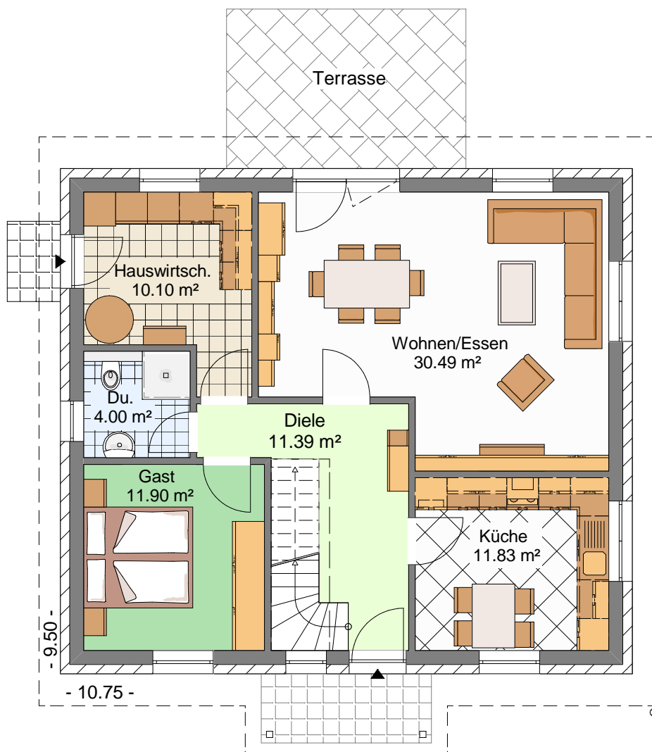
ERDGESCHOSS
