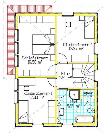
OBERGECHOSS Wohnfläche: 55,26 m 2
