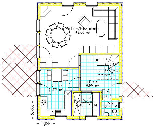
ERDGESCHOSS Wohnfläche: 57,63 m 2
