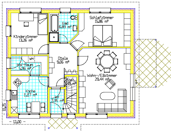
ERDGESCHOSS Wohnung 1 (Wohnfläche: 93,87 m 2 ) Gesamtnutzfläche: 96,81 m 2
