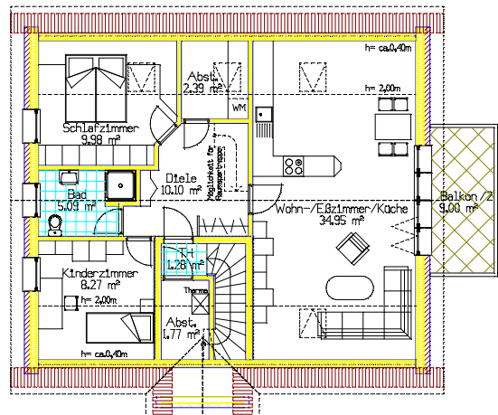
DACHGESCHOSS Wohnung 2 (Wohnfläche: 75,28 m 2 ) Gesamtnutzfläche: 78,33 m 2
