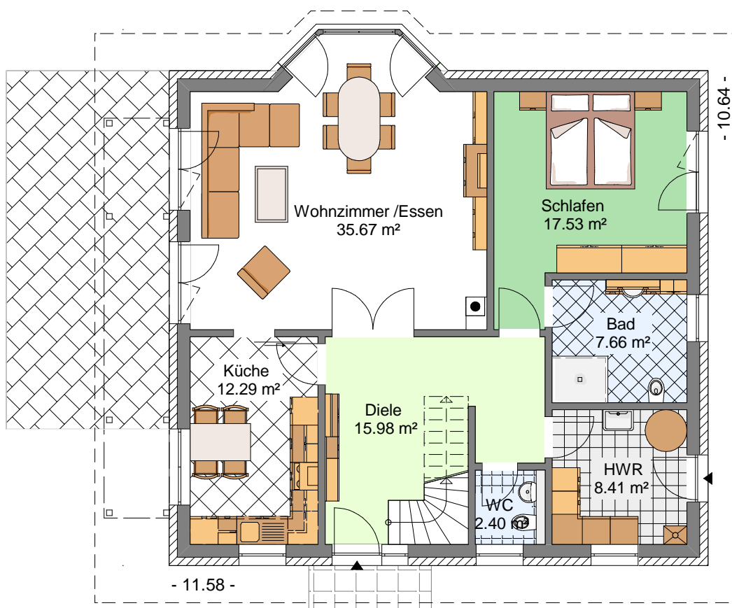
ERDGESCHOSS
