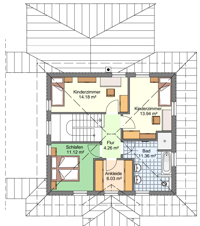
OBERGESCHOSS
