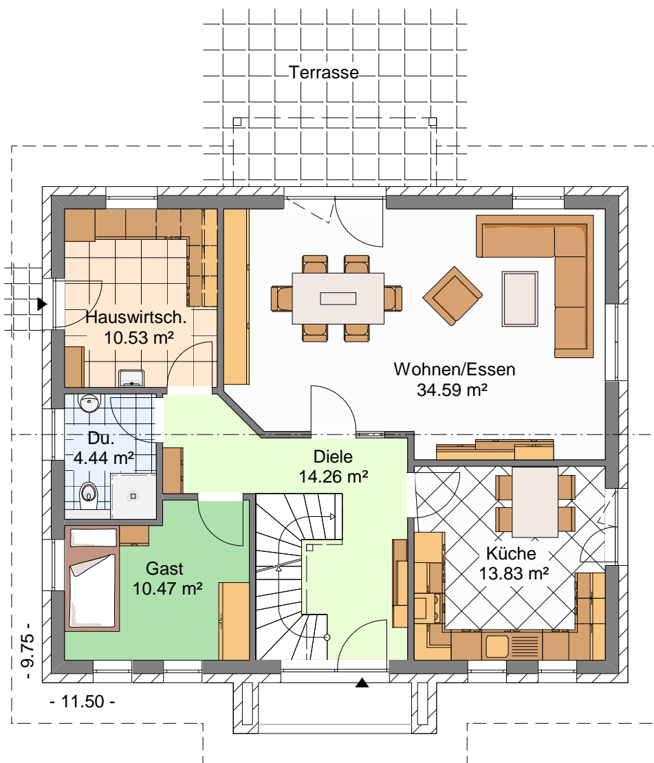
ERDGESCHOSS
