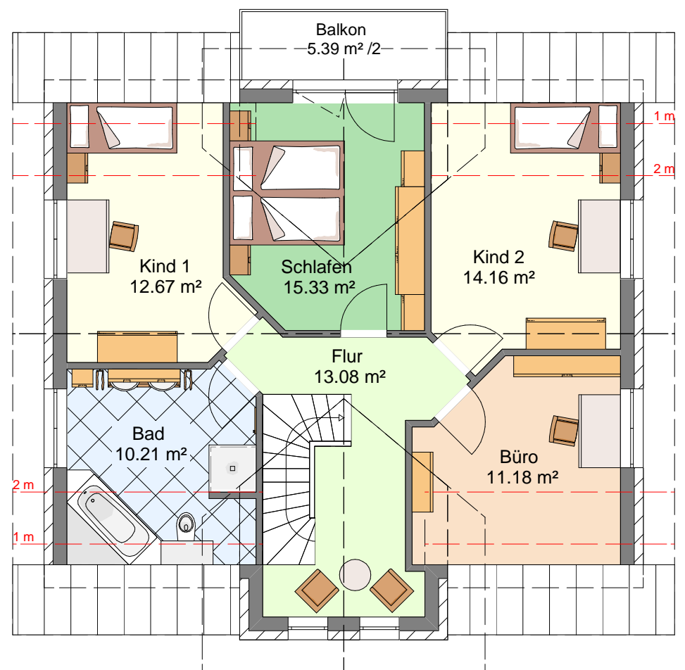
DACHGESCHOSS
